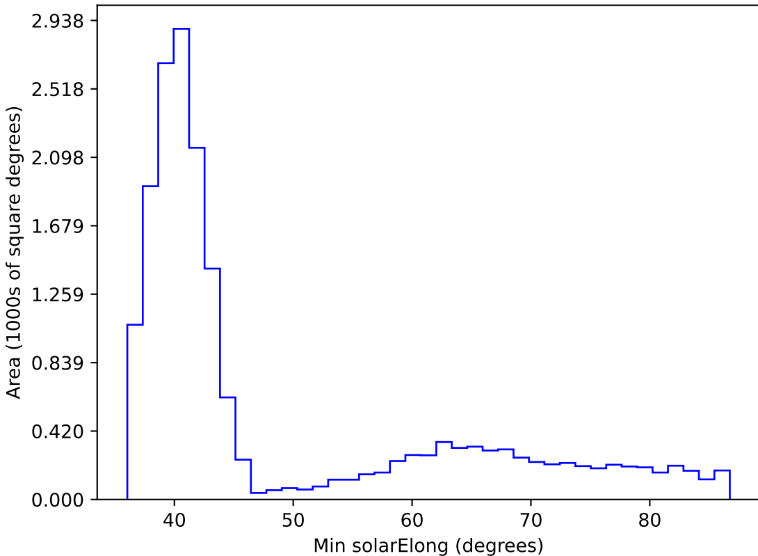
weather_cloudso6v3.4_10yrs WFD i band: Min solarElong
