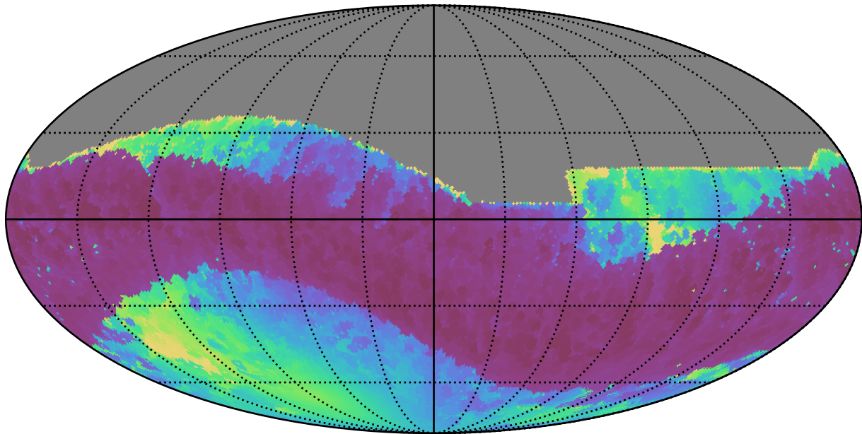
weather_cloudso6v3.4_10yrs All sky z band: Min solarElong
