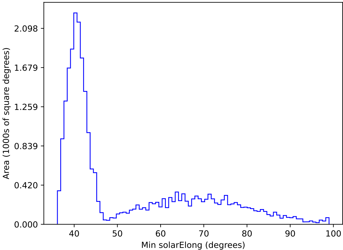
weather_cloudso6v3.4_10yrs All sky z band: Min solarElong
