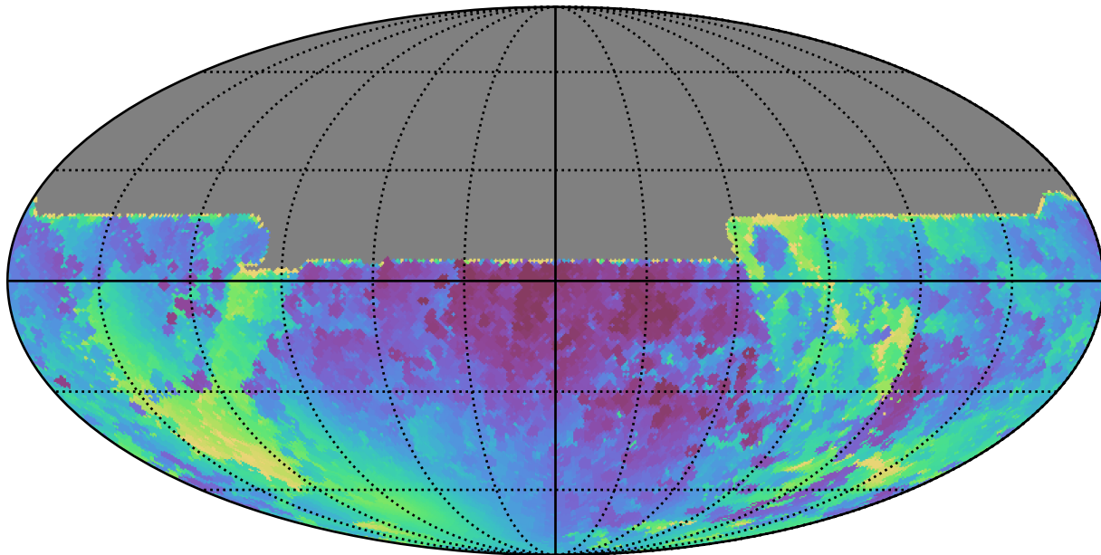
weather_cloudso6v3.4_10yrs All sky y band: Min solarElong
