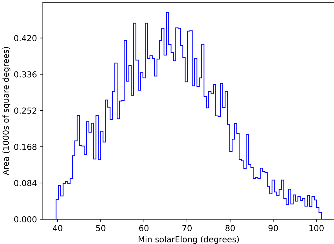
weather_cloudso6v3.4_10yrs All sky y band: Min solarElong
