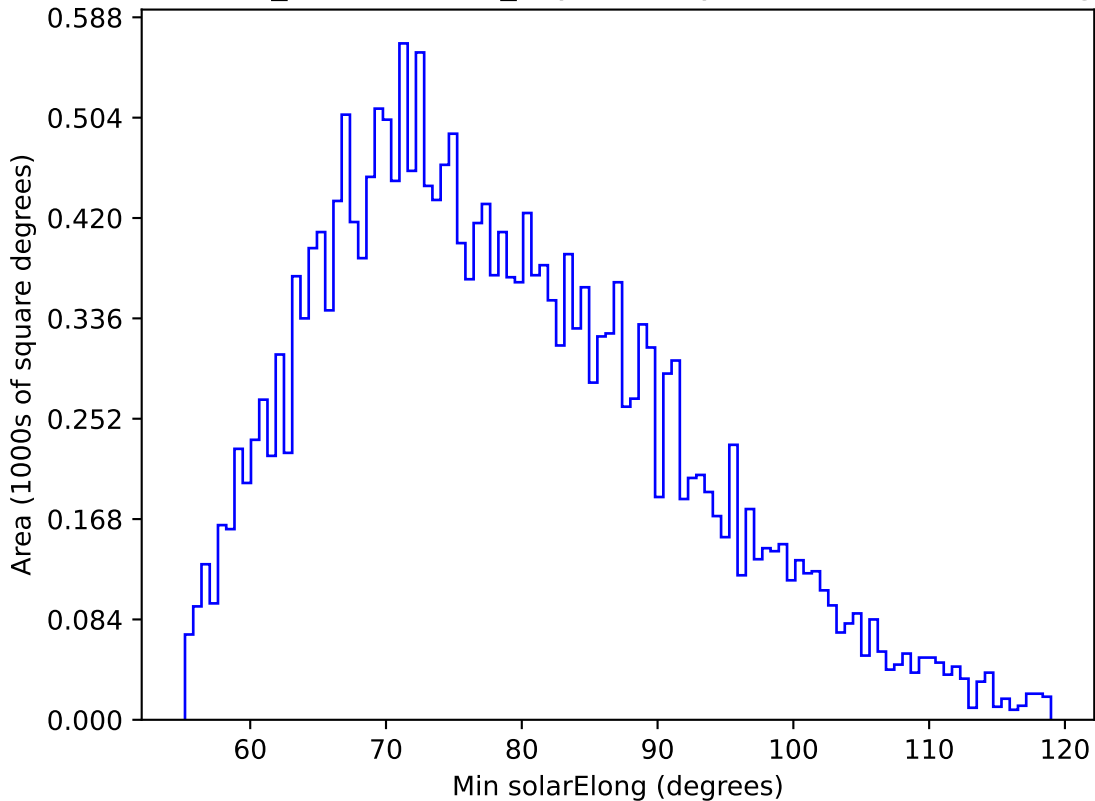
weather_cloudso6v3.4_10yrs All sky u band: Min solarElong
