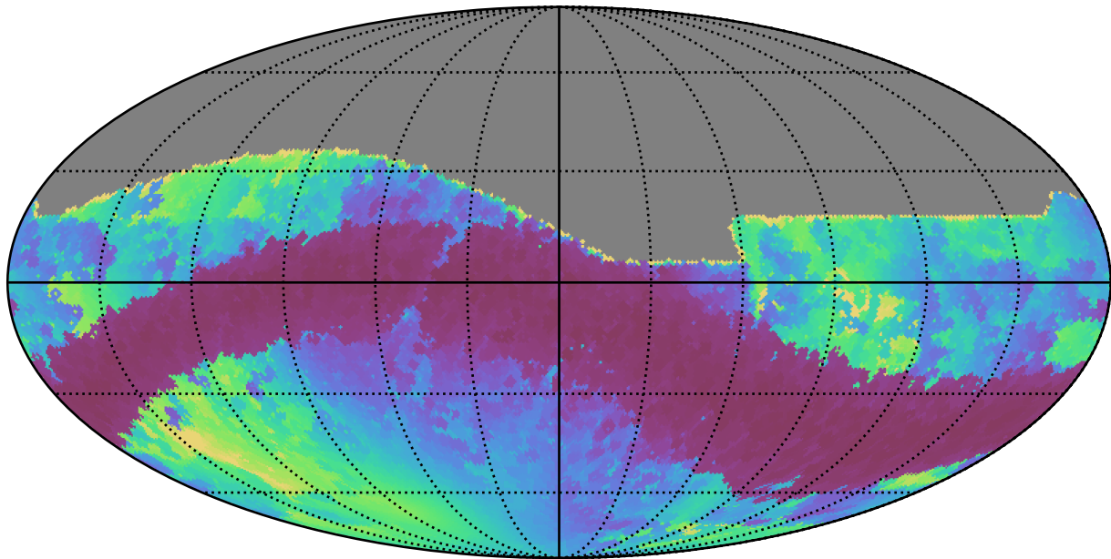
weather_cloudso6v3.4_10yrs All sky r band: Min solarElong
