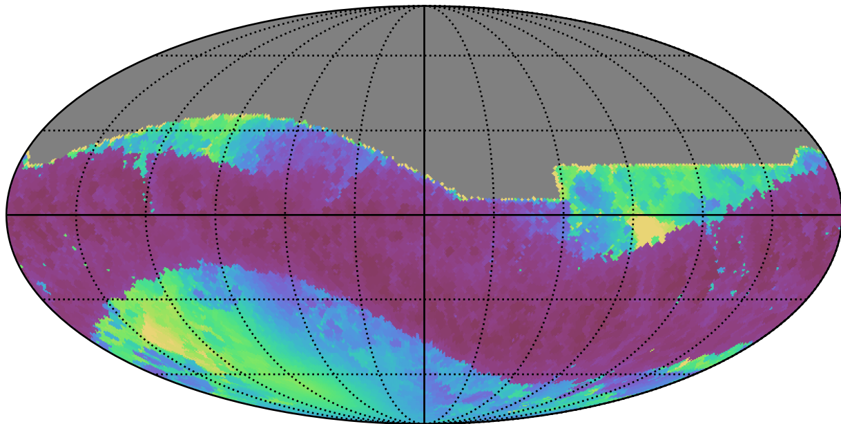
weather_cloudso6v3.4_10yrs All sky i band: Min solarElong
