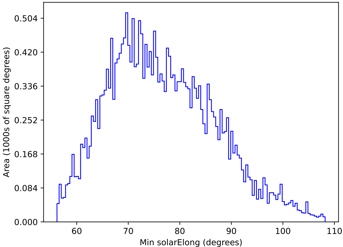
weather_cloudso6v3.4_10yrs All sky g band: Min solarElong
