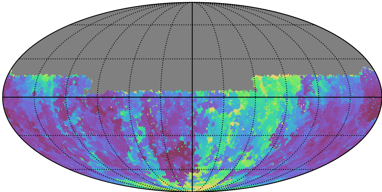
weather_cloudso6v3.4_10yrs Yr 1 u band: Min seeingGeom
