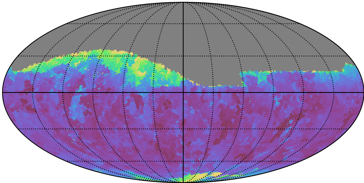
weather_cloudso6v3.4_10yrs Yr 1 r band: Min seeingGeom
