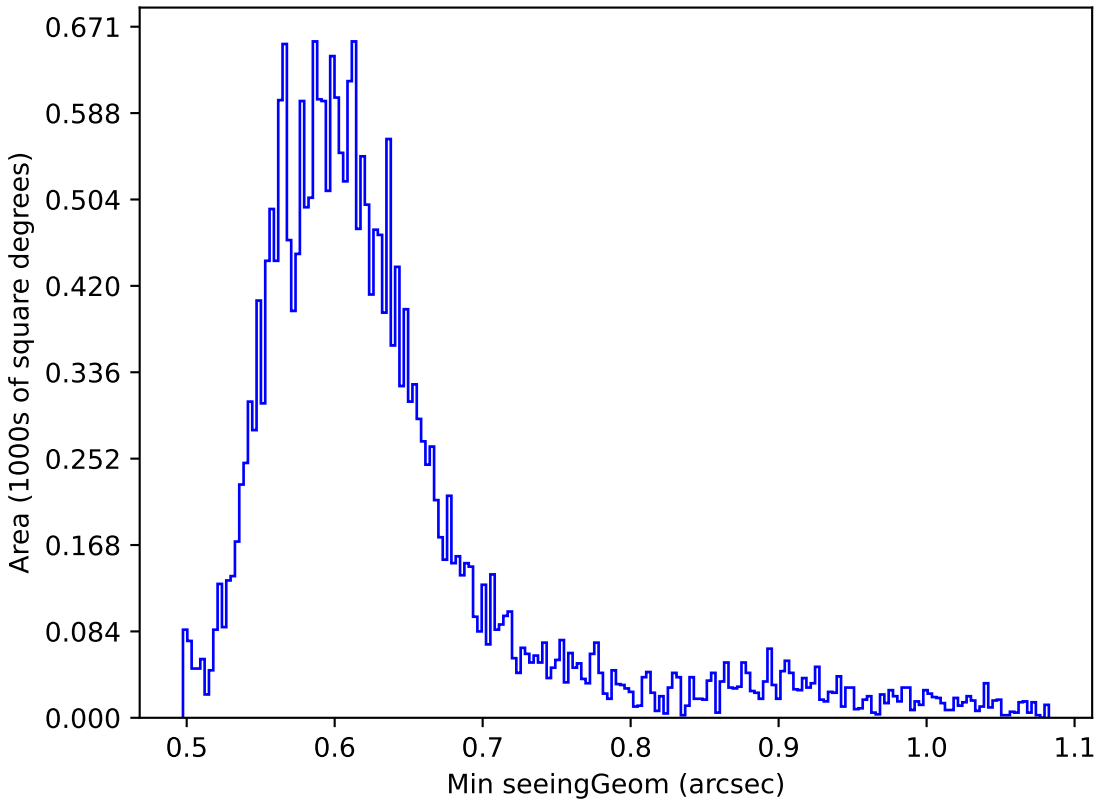
weather_cloudso6v3.4_10yrs Yr 1 r band: Min seeingGeom
