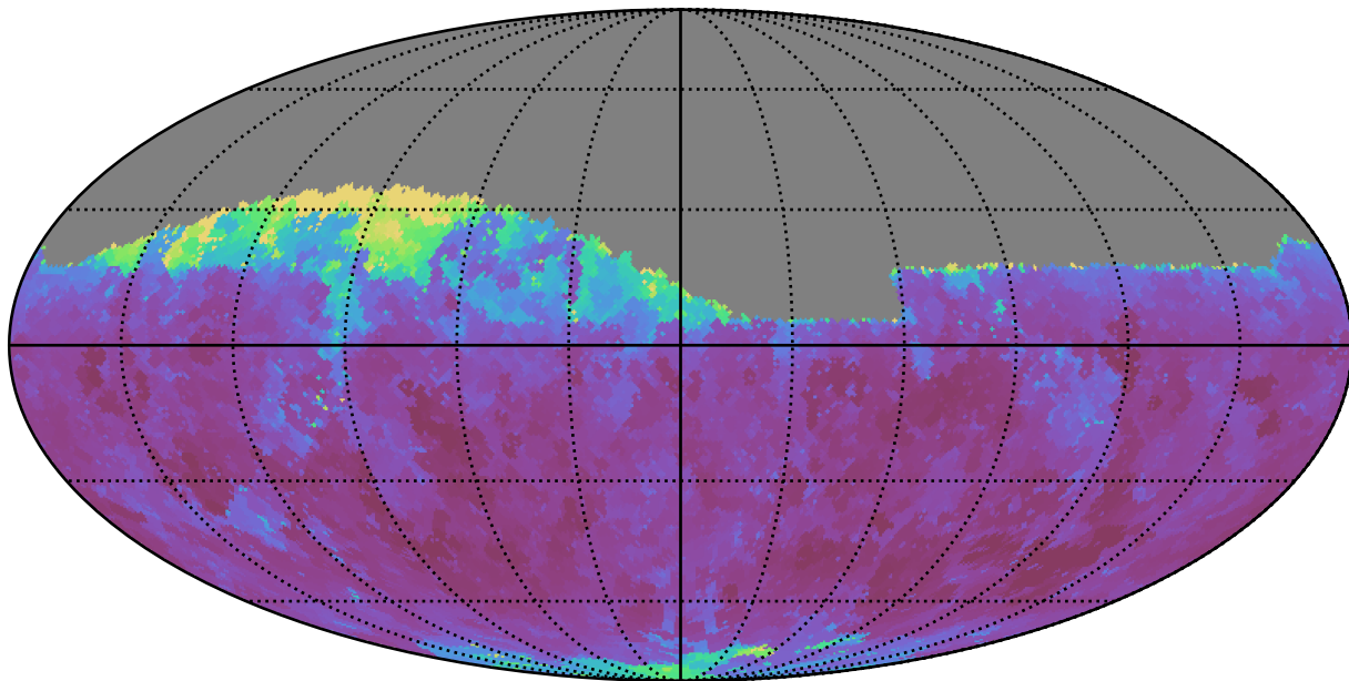
weather_cloudso6v3.4_10yrs Yr 1 i band: Min seeingGeom
