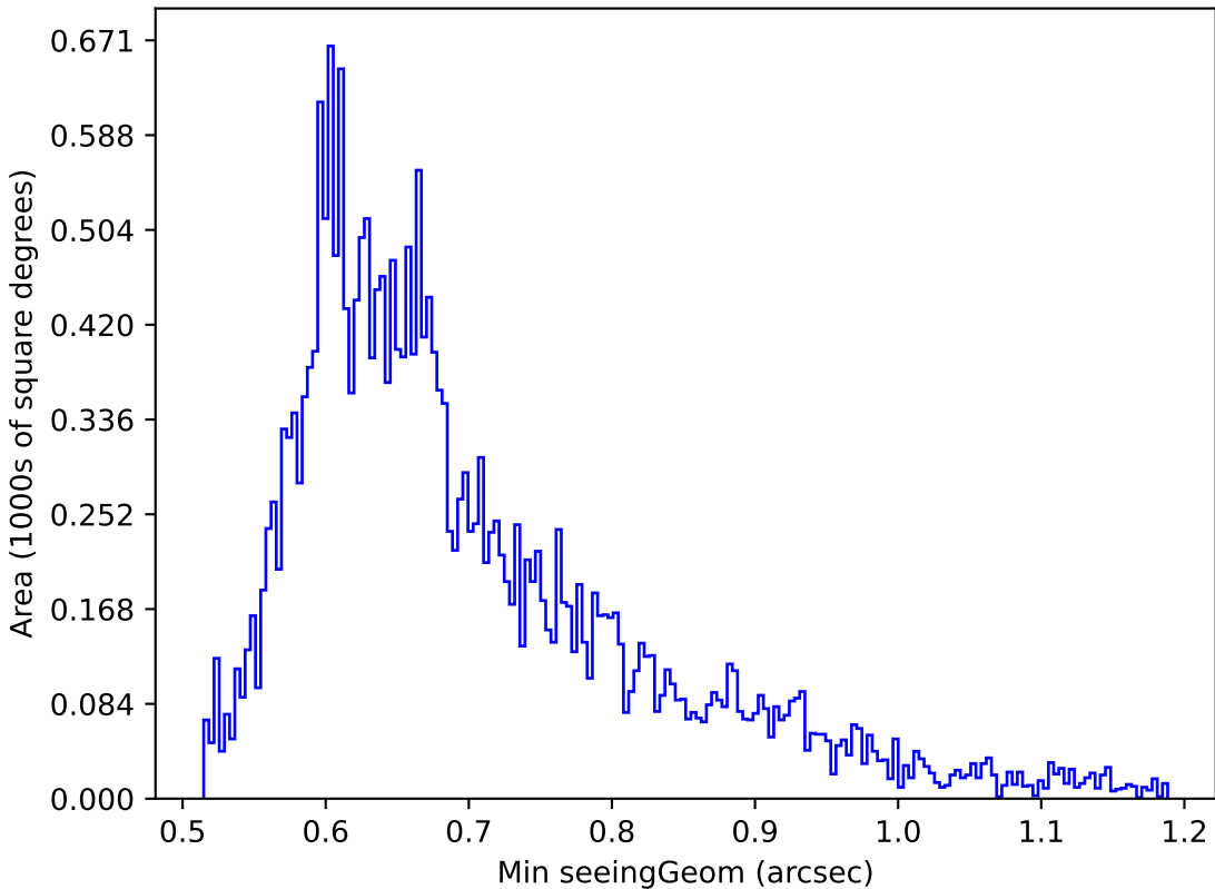
weather_cloudso6v3.4_10yrs Yr 1 g band: Min seeingGeom
