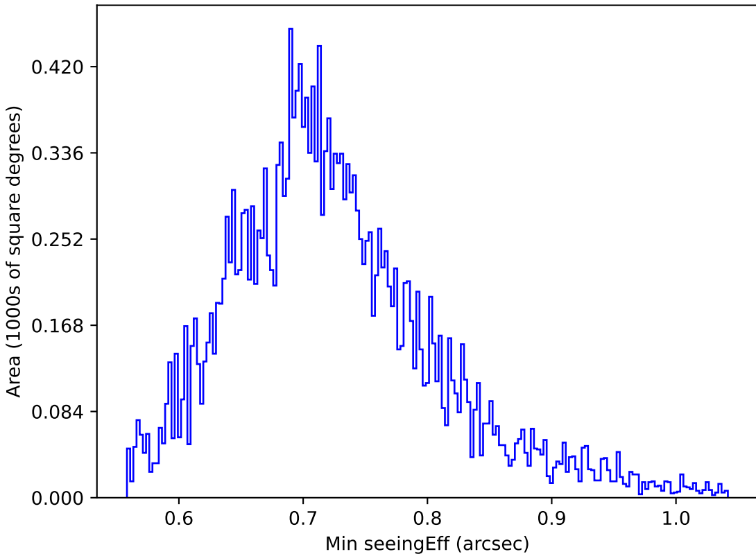
weather_cloudso6v3.4_10yrs Yr 1 y band: Min seeingEff
