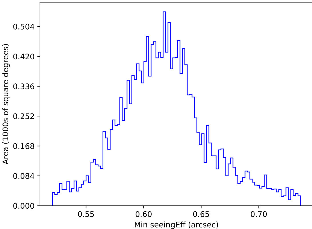
weather_cloudso6v3.4_10yrs WFD z band: Min seeingEff
