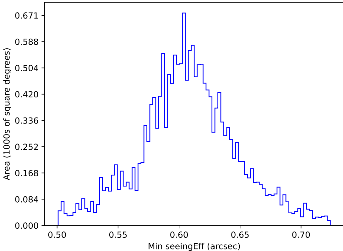
weather_cloudso6v3.4_10yrs WFD i band: Min seeingEff
