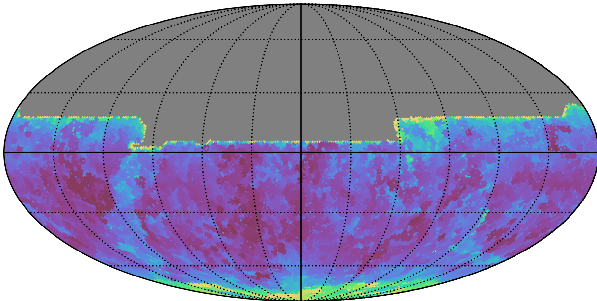
weather_cloudso6v3.4_10yrs All sky y band: Min seeingEff
