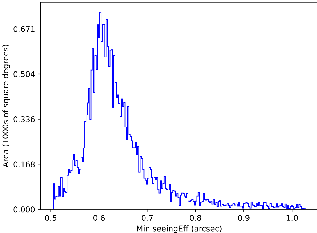
weather_cloudso6v3.4_10yrs All sky i band: Min seeingEff
