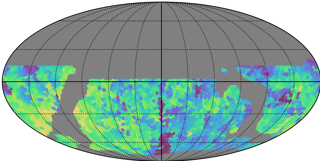
weather_cloudso6v3.4_10yrs WFD z band: Min saturation_mag
