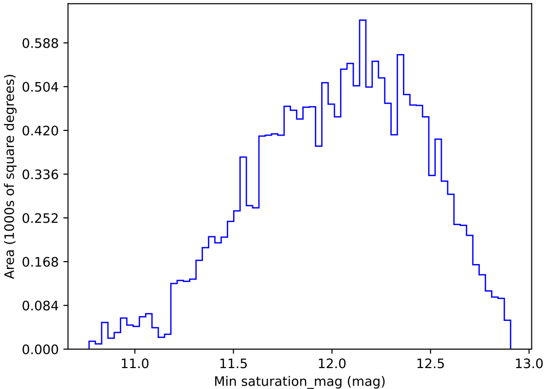
weather_cloudso6v3.4_10yrs WFD z band: Min saturation_mag
