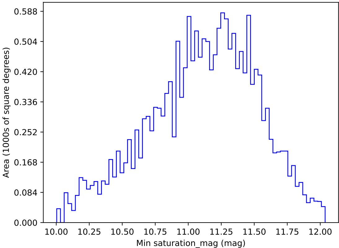
weather_cloudso6v3.4_10yrs WFD y band: Min saturation_mag
