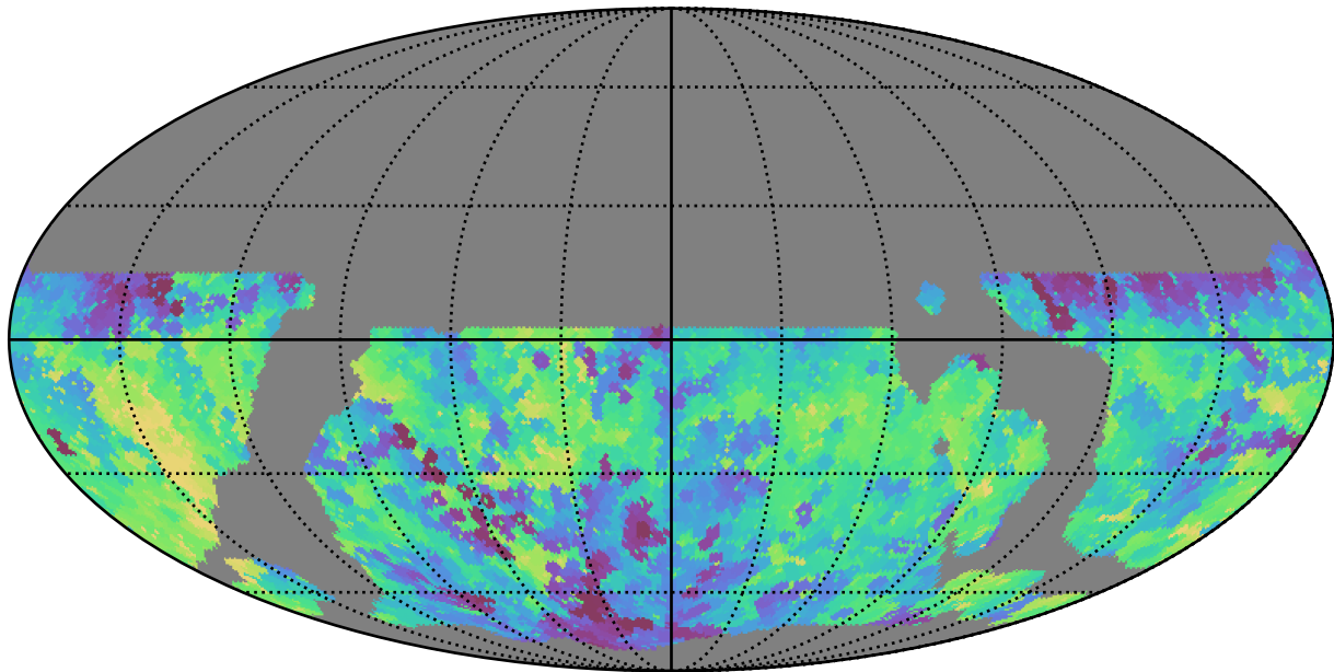
weather_cloudso6v3.4_10yrs WFD u band: Min saturation_mag
