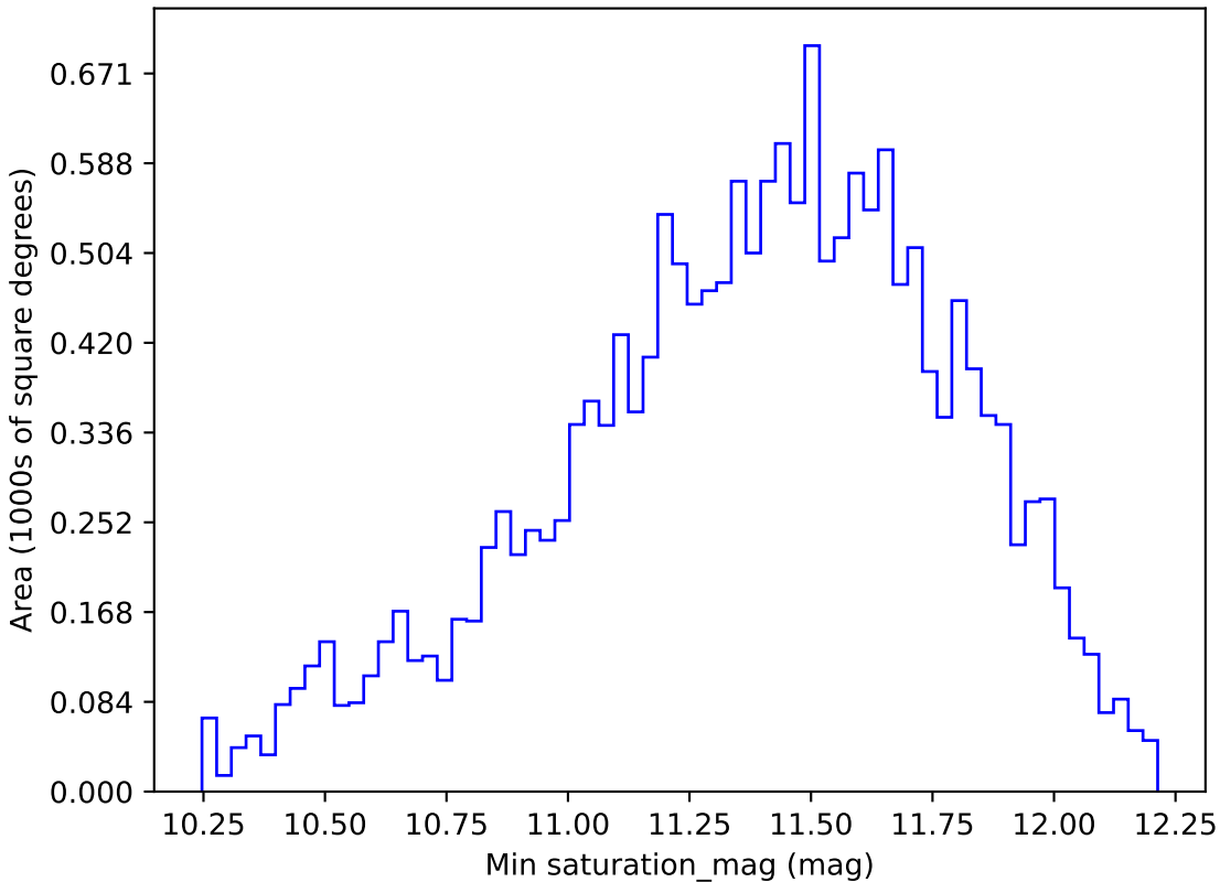
weather_cloudso6v3.4_10yrs WFD u band: Min saturation_mag
