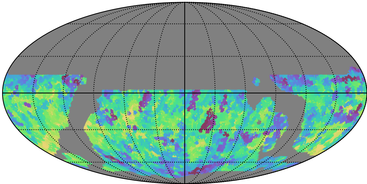
weather_cloudso6v3.4_10yrs WFD r band: Min saturation_mag
