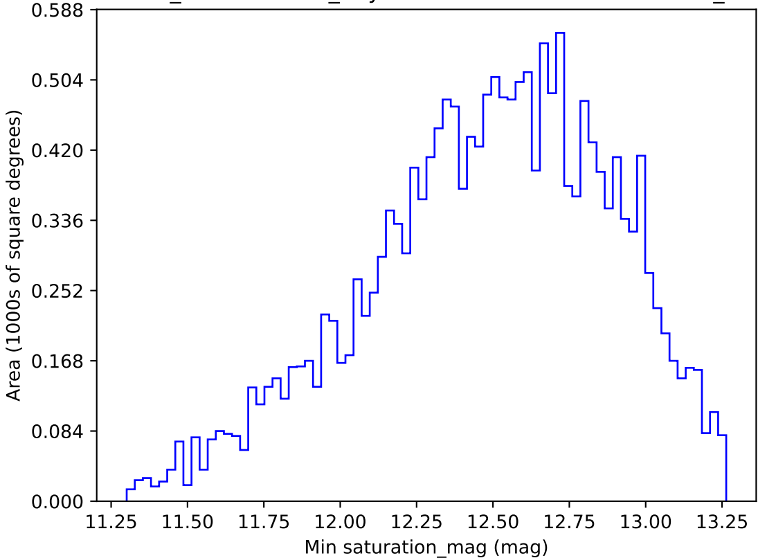
weather_cloudso6v3.4_10yrs WFD r band: Min saturation_mag
