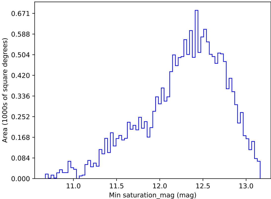
weather_cloudso6v3.4_10yrs WFD i band: Min saturation_mag
