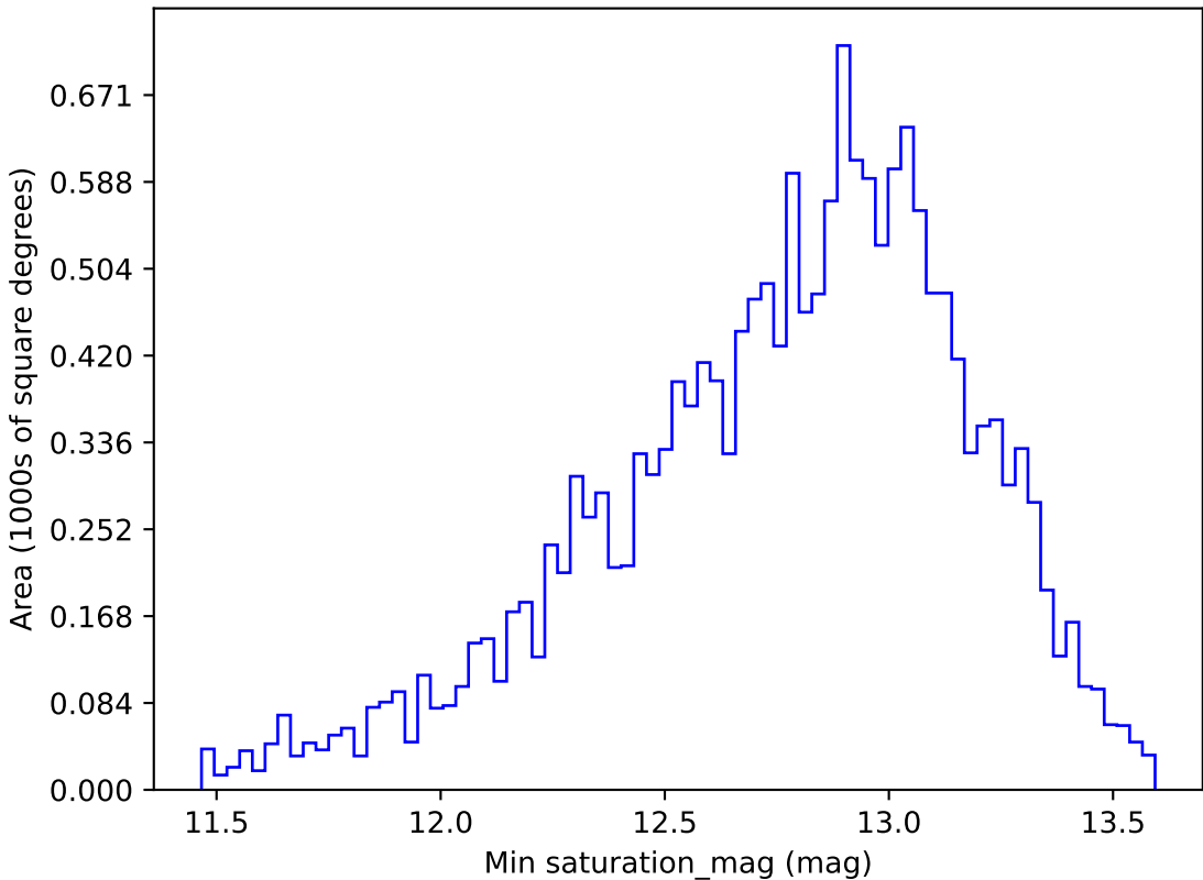
weather_cloudso6v3.4_10yrs WFD g band: Min saturation_mag
