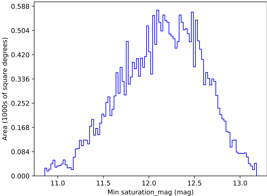
weather_cloudso6v3.4_10yrs All sky z band: Min saturation_mag
