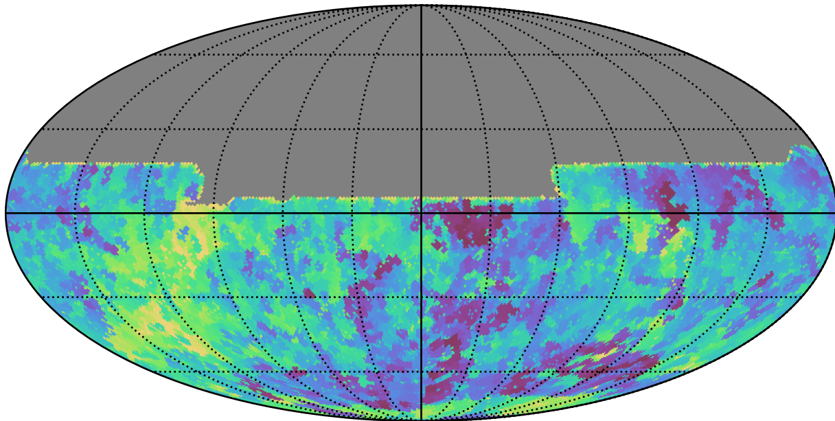
weather_cloudso6v3.4_10yrs All sky y band: Min saturation_mag
