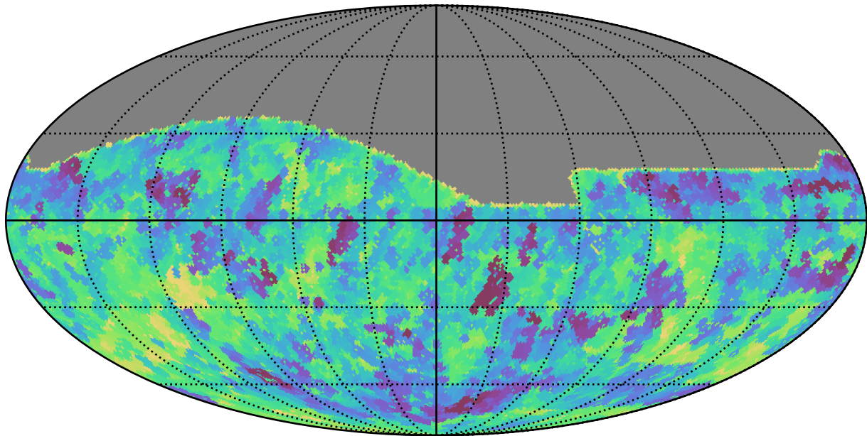
weather_cloudso6v3.4_10yrs All sky r band: Min saturation_mag
