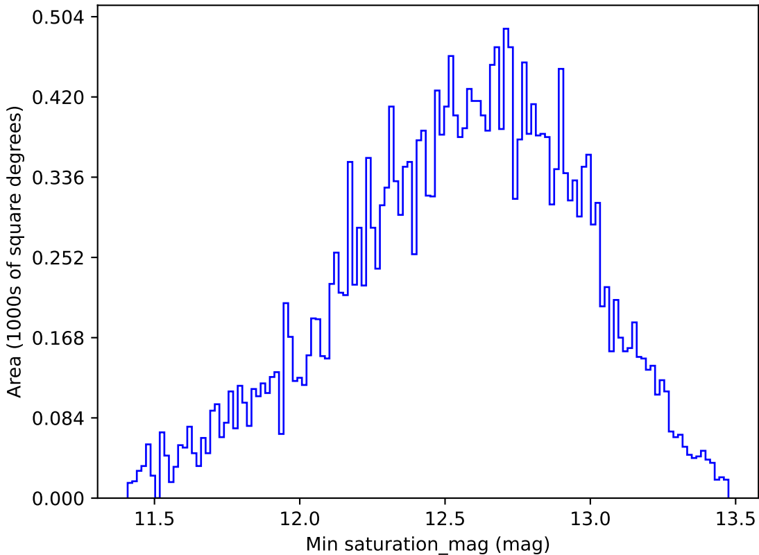
weather_cloudso6v3.4_10yrs All sky r band: Min saturation_mag
