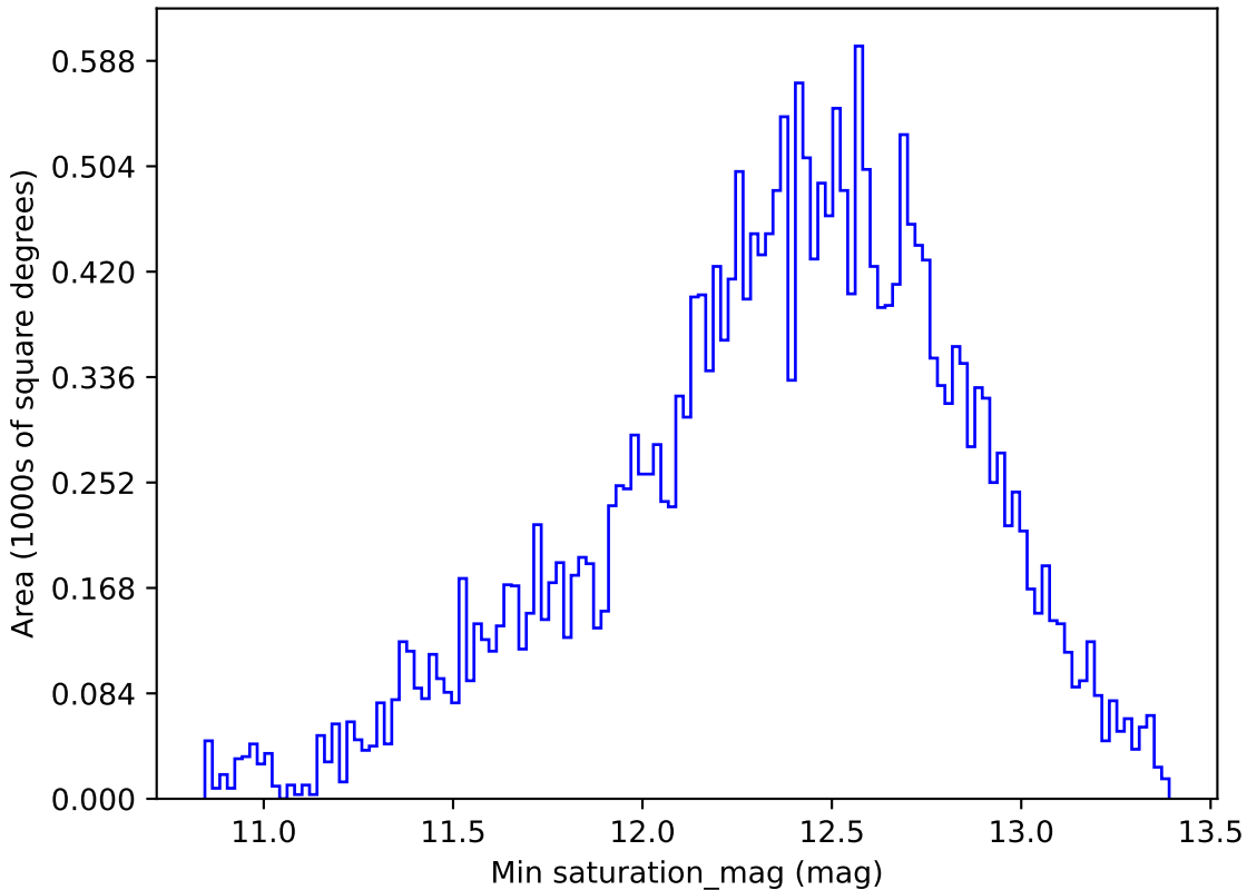
weather_cloudso6v3.4_10yrs All sky i band: Min saturation_mag
