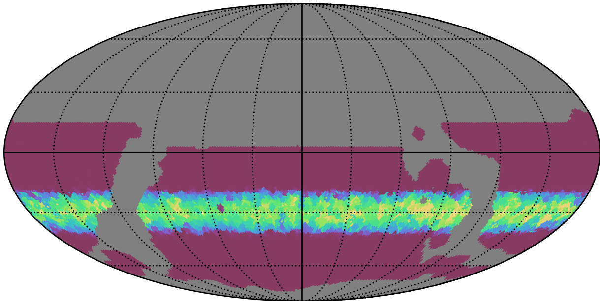
weather_cloudso6v3.4_10yrs WFD z band: Min normairmass
