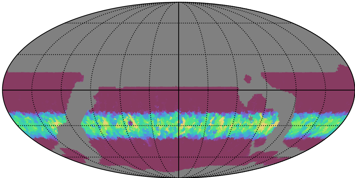
weather_cloudso6v3.4_10yrs WFD u band: Min normairmass
