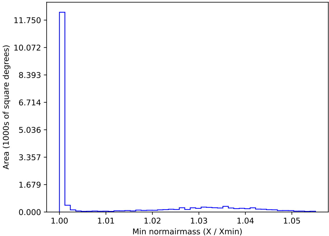
weather_cloudso6v3.4_10yrs WFD u band: Min normairmass
