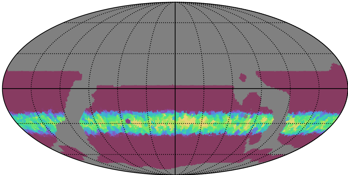
weather_cloudso6v3.4_10yrs WFD r band: Min normairmass
