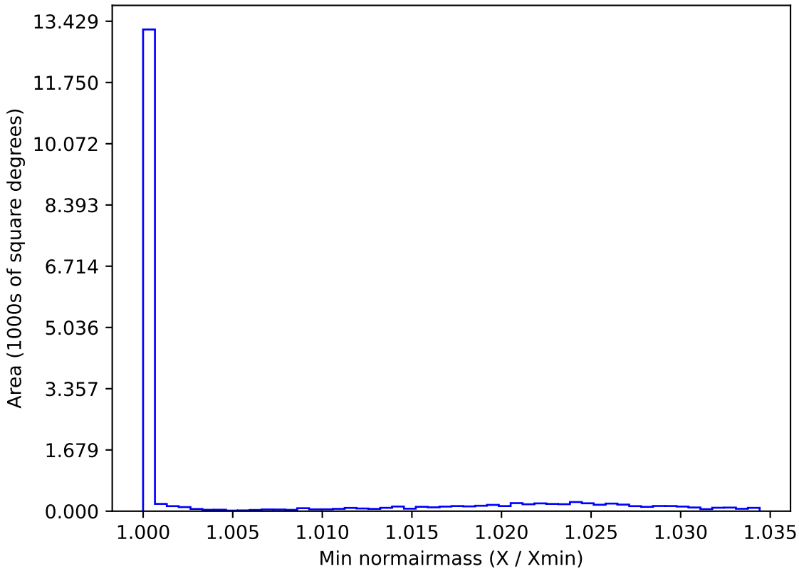
weather_cloudso6v3.4_10yrs WFD r band: Min normairmass
