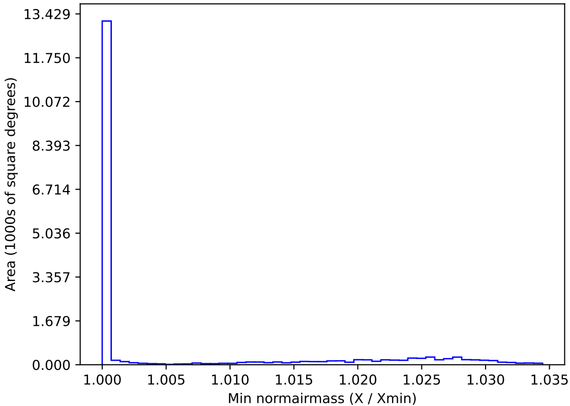
weather_cloudso6v3.4_10yrs WFD i band: Min normairmass
