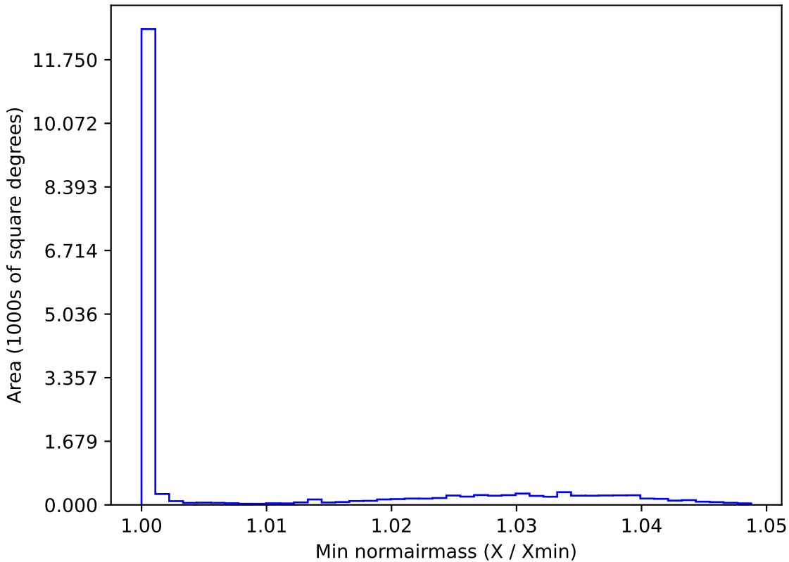
weather_cloudso6v3.4_10yrs WFD g band: Min normairmass
