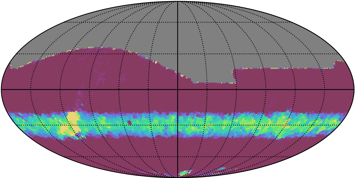
weather_cloudso6v3.4_10yrs All sky z band: Min normairmass
