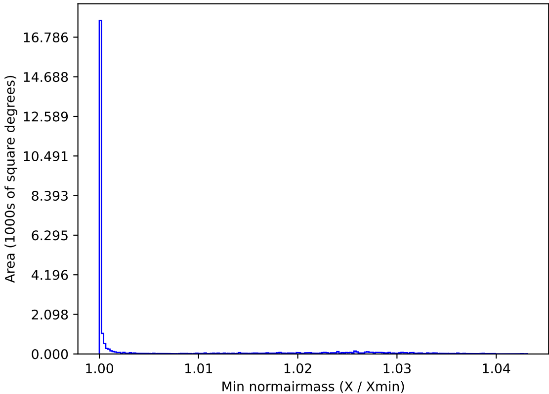
weather_cloudso6v3.4_10yrs All sky z band: Min normairmass
