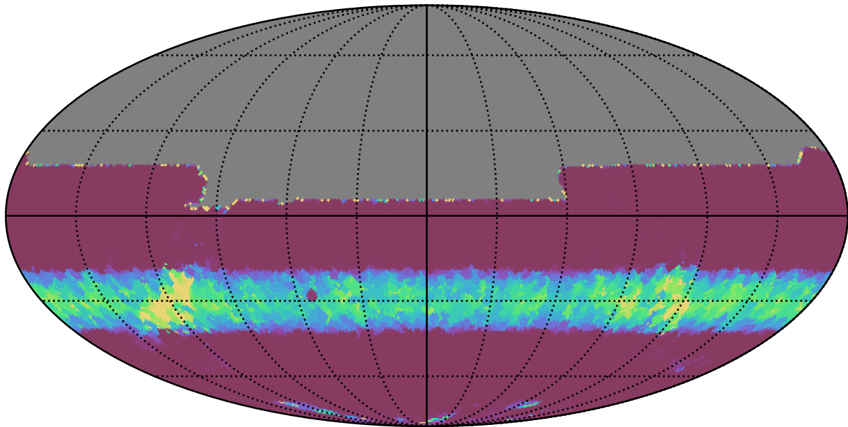
weather_cloudso6v3.4_10yrs All sky y band: Min normairmass
