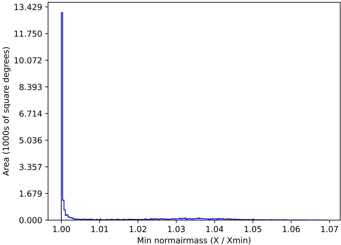
weather_cloudso6v3.4_10yrs All sky u band: Min normairmass
