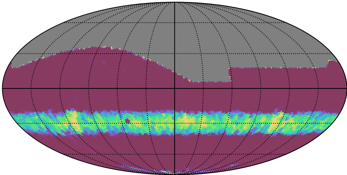
weather_cloudso6v3.4_10yrs All sky r band: Min normairmass
