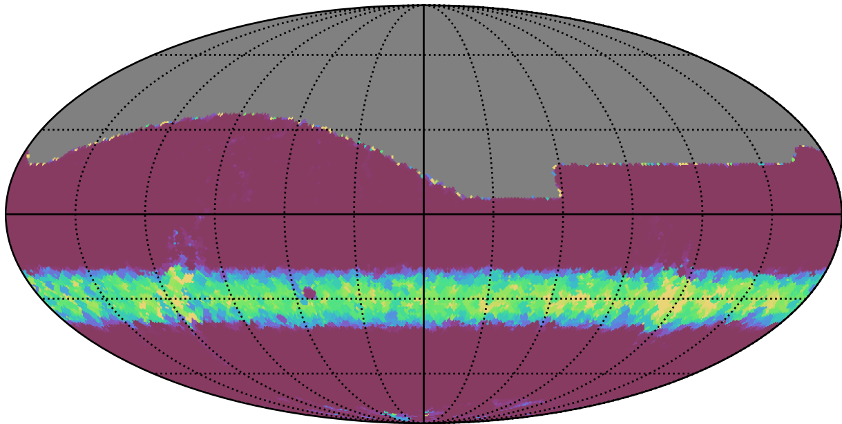
weather_cloudso6v3.4_10yrs All sky i band: Min normairmass
