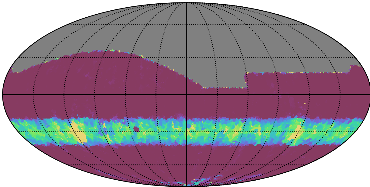
weather_cloudso6v3.4_10yrs All sky g band: Min normairmass
