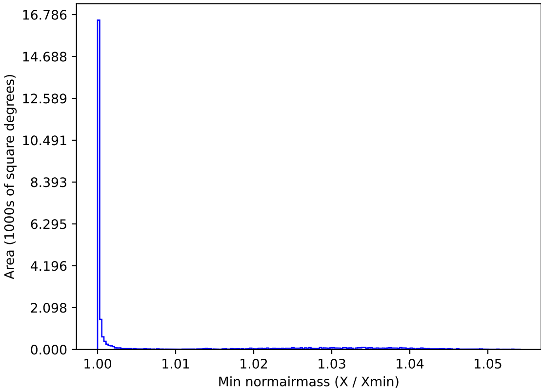
weather_cloudso6v3.4_10yrs All sky g band: Min normairmass
