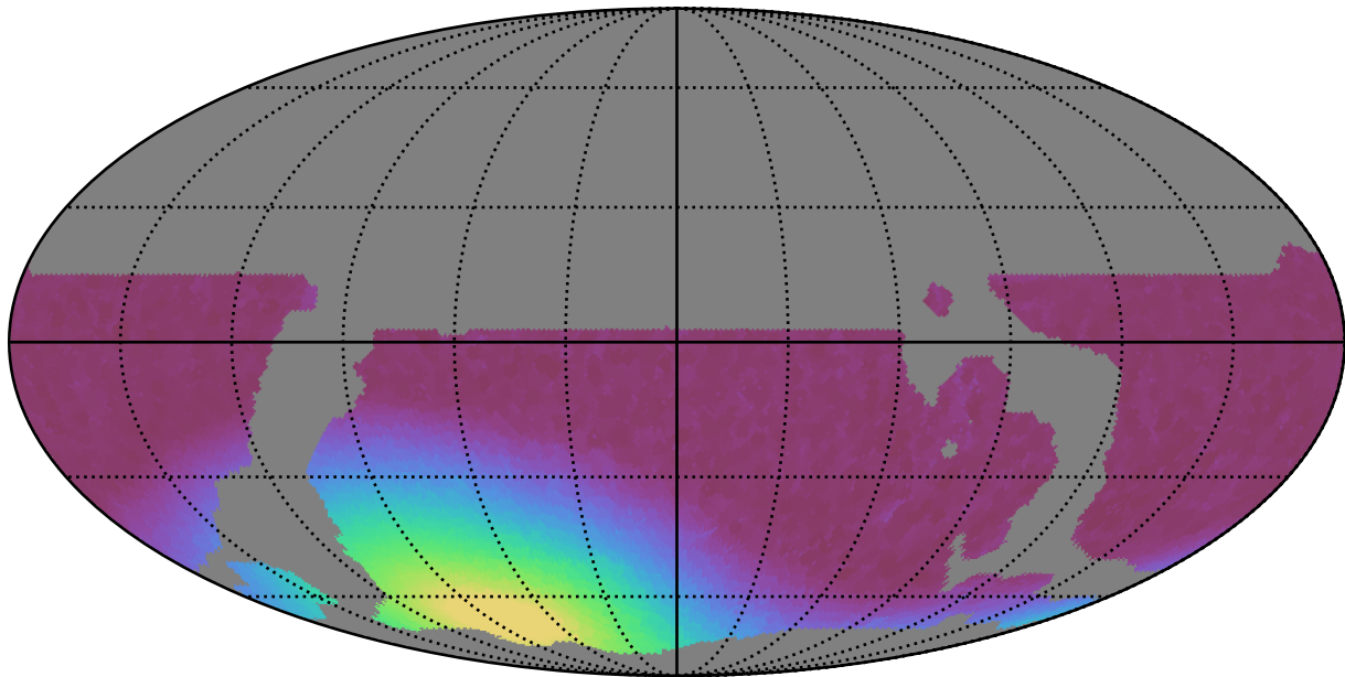
weather_cloudso6v3.4_10yrs WFD z band: Min moonDistance
