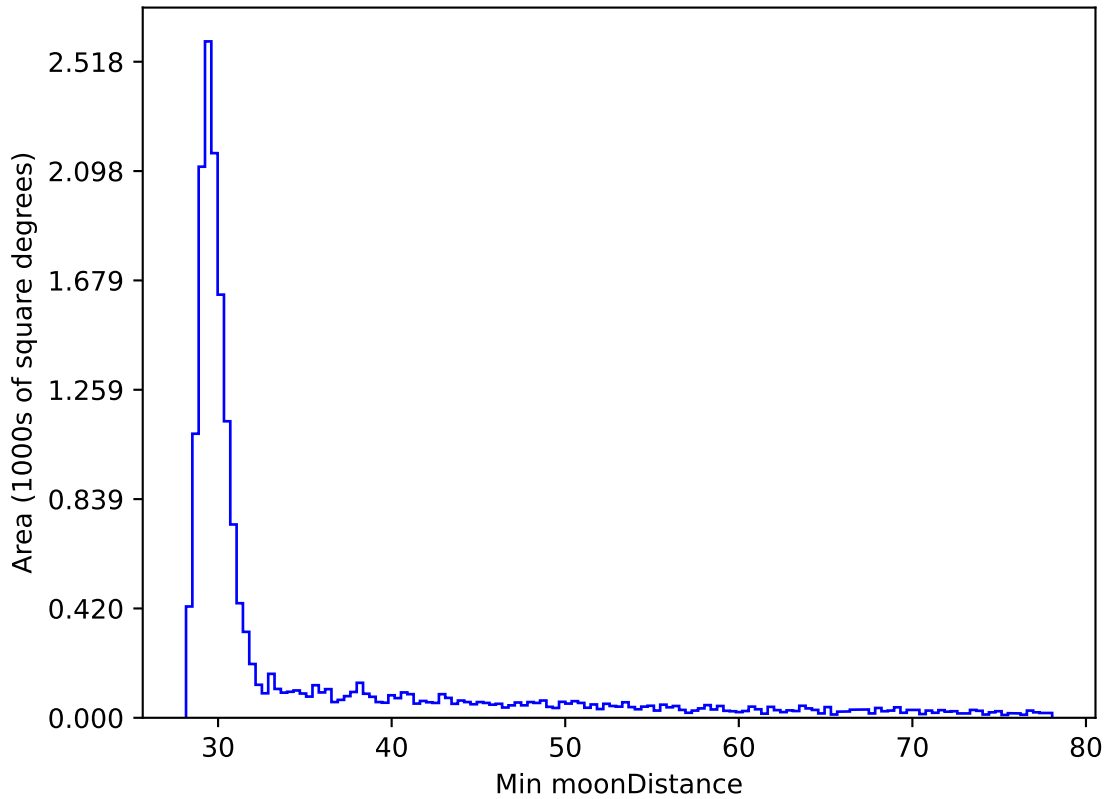
weather_cloudso6v3.4_10yrs WFD z band: Min moonDistance
